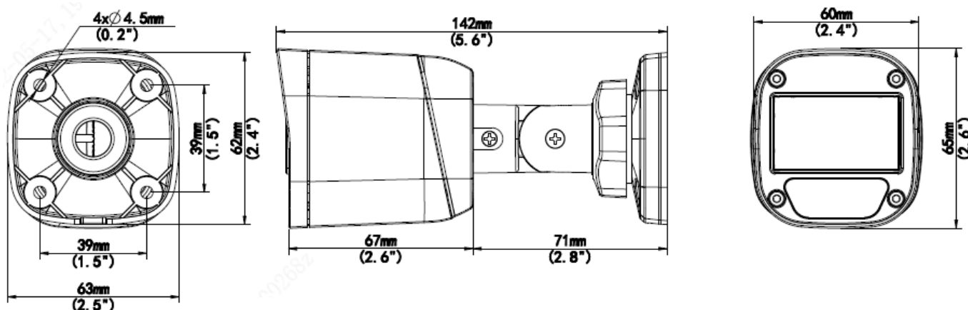
UAC-B1A15(2.8/4.0mm)
